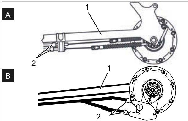
Figura 170: Casquillos de ajuste (2) en dos versiones alternativas (A y B) de un cambio de marchas accionado por cable de accionamiento, de dos cables en la vaina (1)
