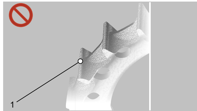
Figura 157: Perfil dentado desgastado
