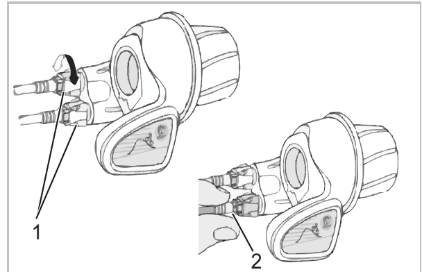
Figura 171: Puño giratorio con casquillos de ajuste (1) con holgura de giro (2)
