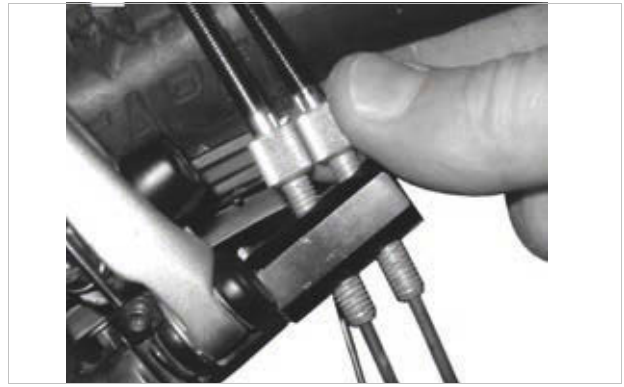
Figura 168: Las versiones de bujes ROHLOFF con activación de cambio interna tienen los dispositivos de ajuste de tensión en el contraapoyo de tensión
