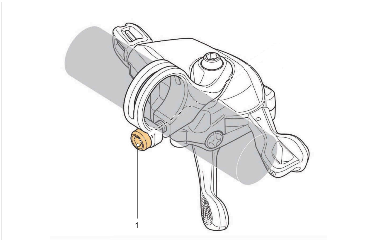
Figura 90: Posición del tornillo de fijación de la palanca de cambio SHIMANO (1)
