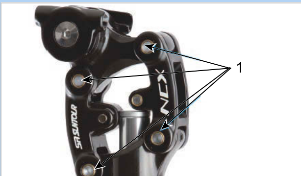
Figura 174: Puntos de lubricación de la tija de sillín de muelle SR SUNTOUR
