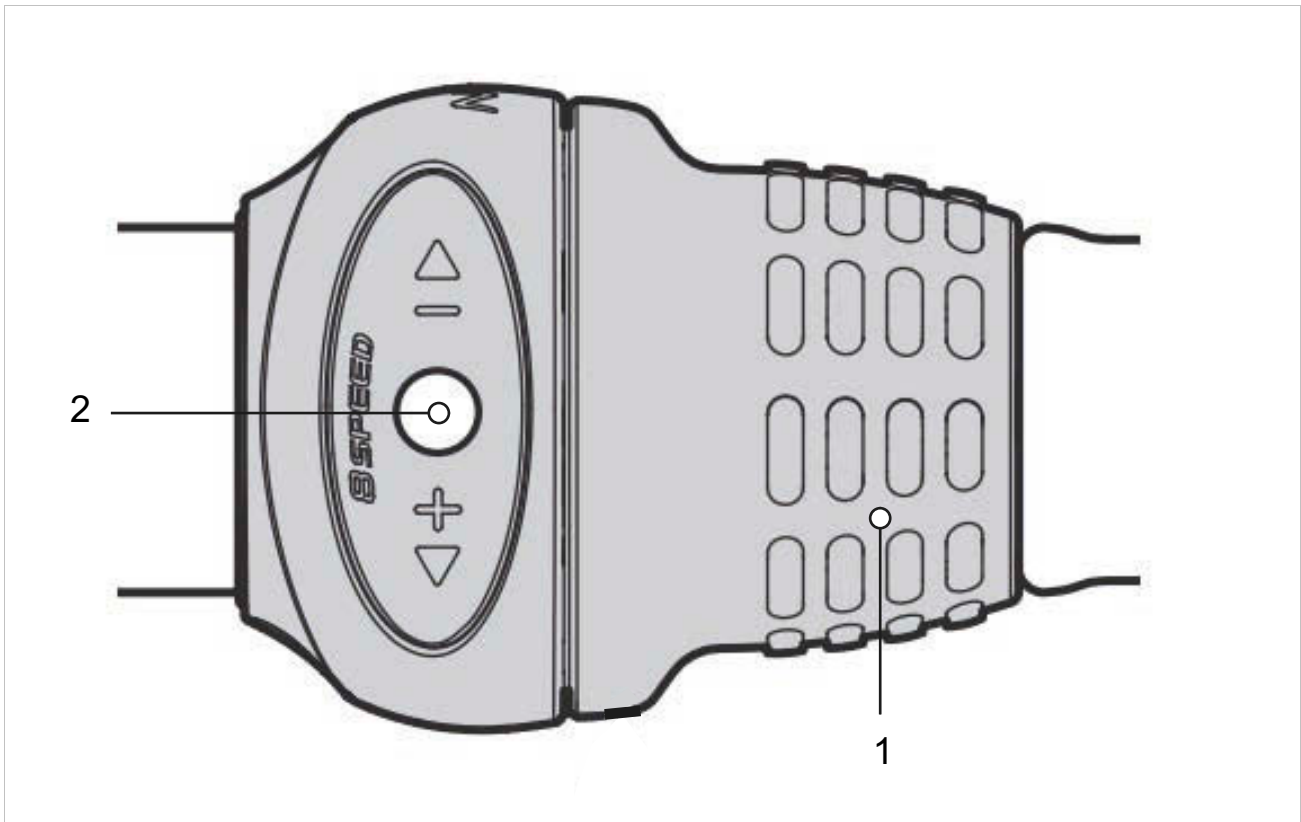
Figura 44: Puño giratorio SHIMANO SL-C30000-7, vista desde arriba
