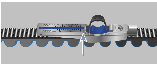
Figura 160: Calibre de comprobación en la correa
