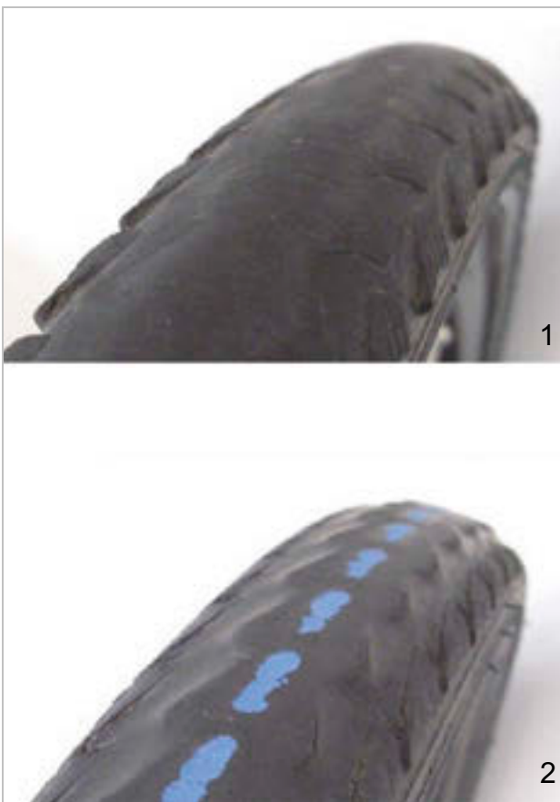
Figura 142: Cubierta sin perfil que puede cambiarse (1); cubierta con protección contra pinchazos visible (2) que tiene que cambiarse
