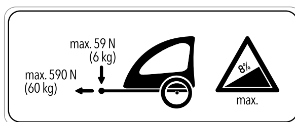
Figura 100: Placa indicadora de remolque
