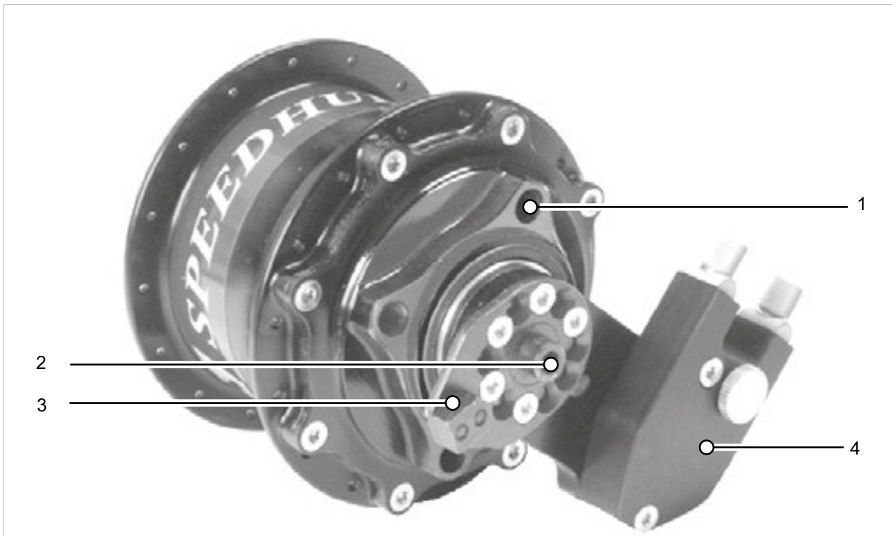
Figura 49: Datos técnicos y funciones de ROHLOFF, Speedhub 500/14 CC DB OEM, black, 32 holes, con tapa del disco de freno (1), eje de cierre rápido (2), placa de trabajo CC OEM (3) y activación de cambio externa (4)
