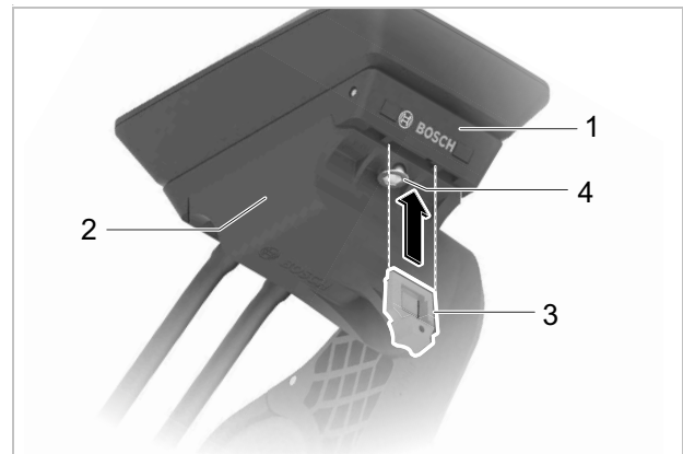
Figura 96: Posición del tornillo del juego de dirección
