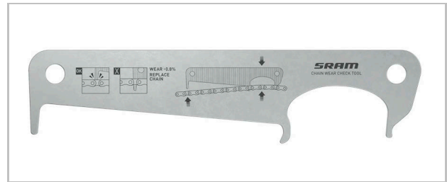
Figura 148: Ejemplo de calibre de medición SRAM
