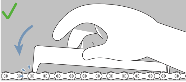
Figura 153: El calibre de medición no cabe
