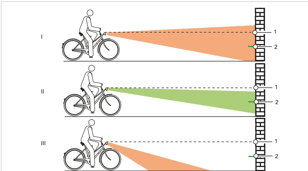
Figura 94: Luz ajustada demasiado alta (1), correctamente (2) y demasiado baja (3)
