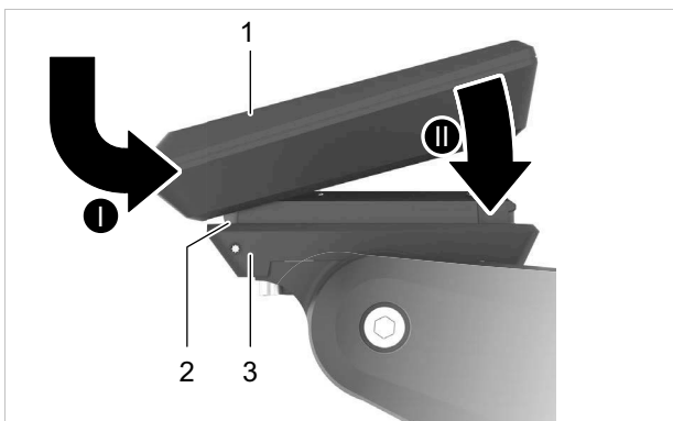
Figura 95: Inserción de la pantalla
