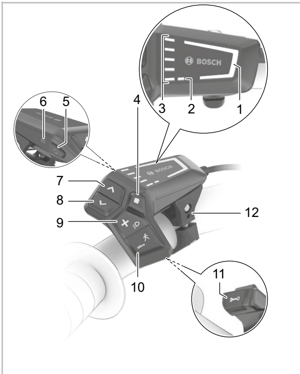
Figura 124: Vista general del ordenador de a bordo BOSCH LED Remote
