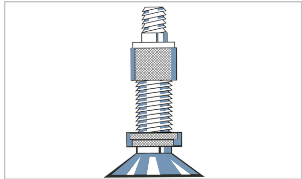
Figura 15: Válvula Dunlop
