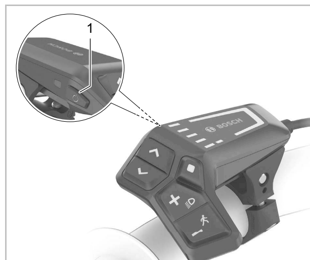
Figura 123: Posición del botón de conexión/desconexión en la BOSCH LED Remote
