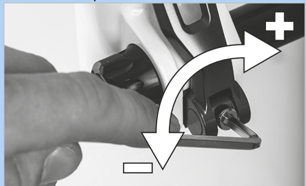
Figura 173: Ajuste de la fuerza de tensado del cierre rápido
