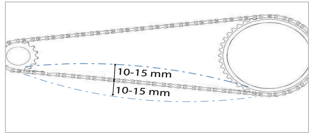
Figura 145: Ejemplo de comprobación de la tensión de la cadena: 5 mm hacia arriba, 10 mm hacia abajo = 15 mm de diferencia
