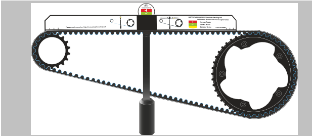
Figura 164: Regla colocada
