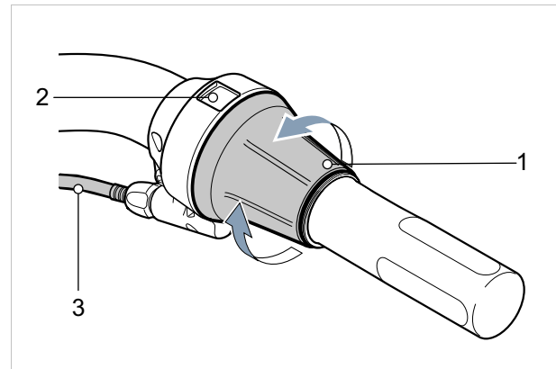
Figura 132: Cambio de marchas SHIMANO SL-C30000-70
