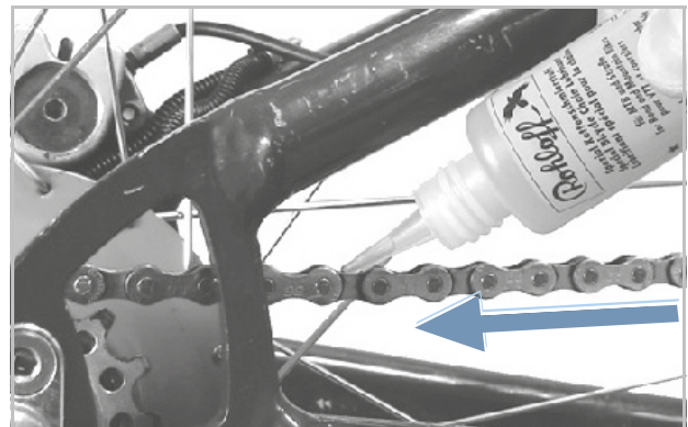
Figura 139: Lubricar cadena
