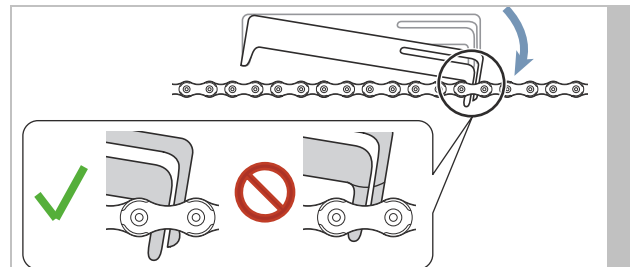
Figura 151: El calibre de medición se inserta
