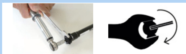
Figura 133: Ajuste en sentido horario
