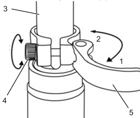
Figura 46: Apertura del cierre rápido de la tija de sillín
