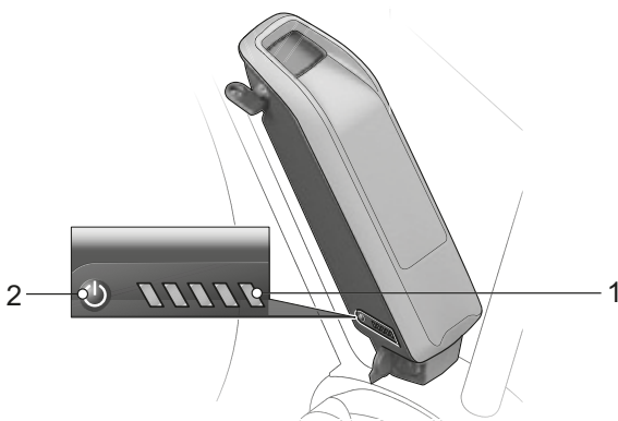
Figura 34: Posición del indicador de carga de la batería en el tubo del sillín
