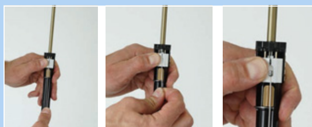
Figura 116: Desenganchar el cable de accionamiento
