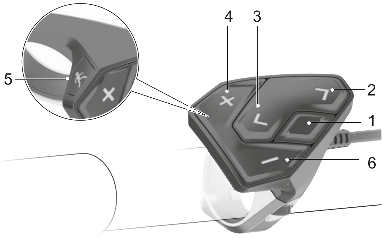
Figura 30: Vista general de la unidad de mando BOSCH
