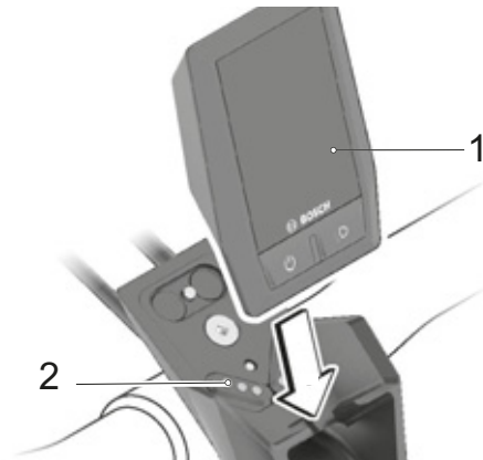
Figura 70: Colocación del ordenador de a bordo (1)
