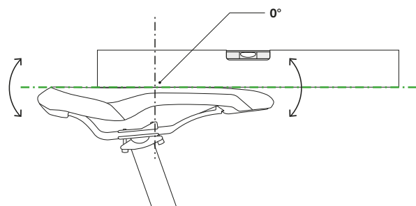
Figura 50: Inclinación del sillín horizontal con 0° de inclinación en el centro del sillín
