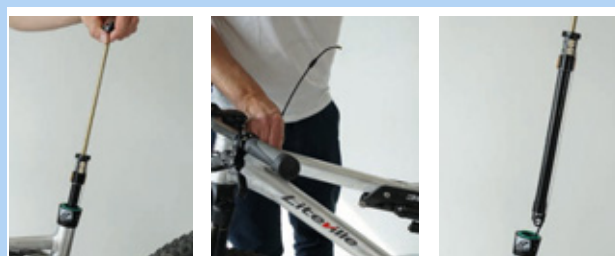
Figura 115: Extracción del cartucho
