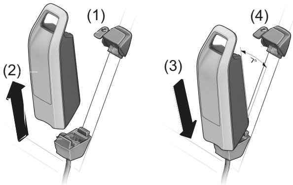
Figura 83: Extracción e inserción de la batería en el cuadro
