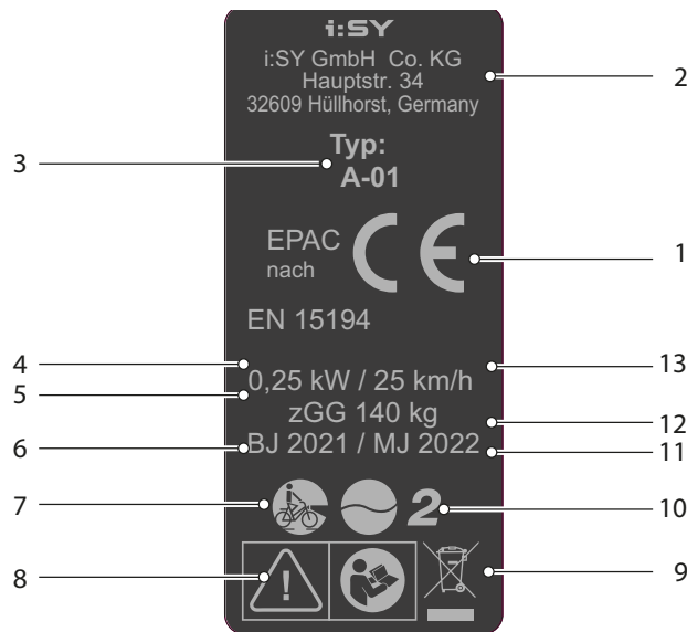
Figura 1: Ejemplo Placa indicadora de tipo i:SY
