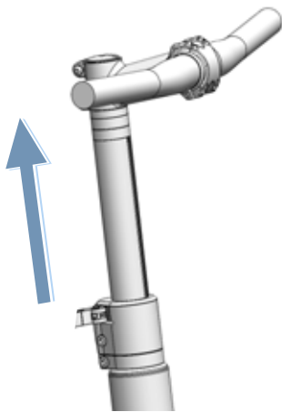
Figura 92: Ejemplo de All Up estirado hasta la posición más alta
