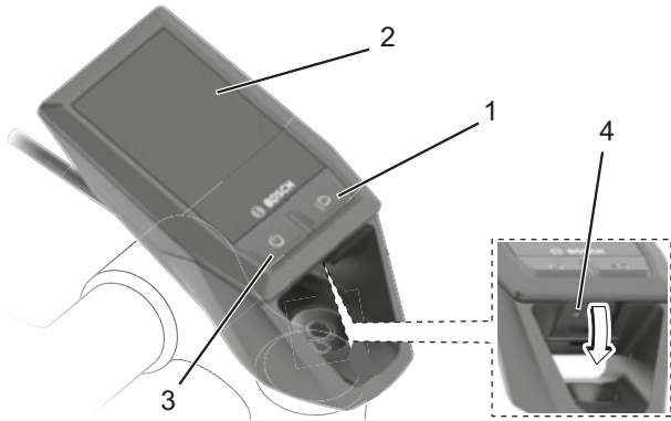
Figura 69: Vista general de la estructura y los elementos de mando del ordenador de a bordo
