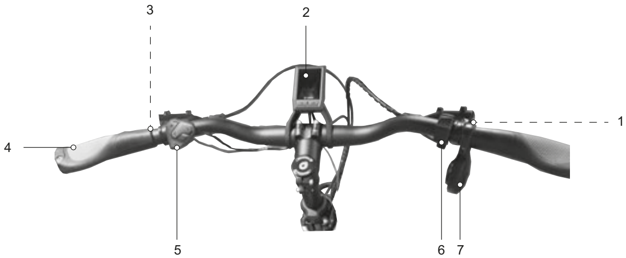
Figura 26: Vista detallada del manillar con ordenador de a bordo BOSCH Kiox, ejemplo
