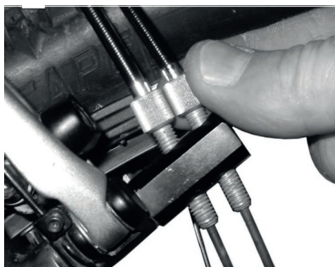
Abbildung 92: ROHLOFF-Naben Versionen mit interner Schaltansteuerung haben die Zugeinsteller am Zuggegenhalter
