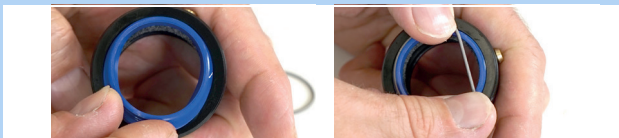
Abbildung 113: Abstreifer einlegen und befestigen
