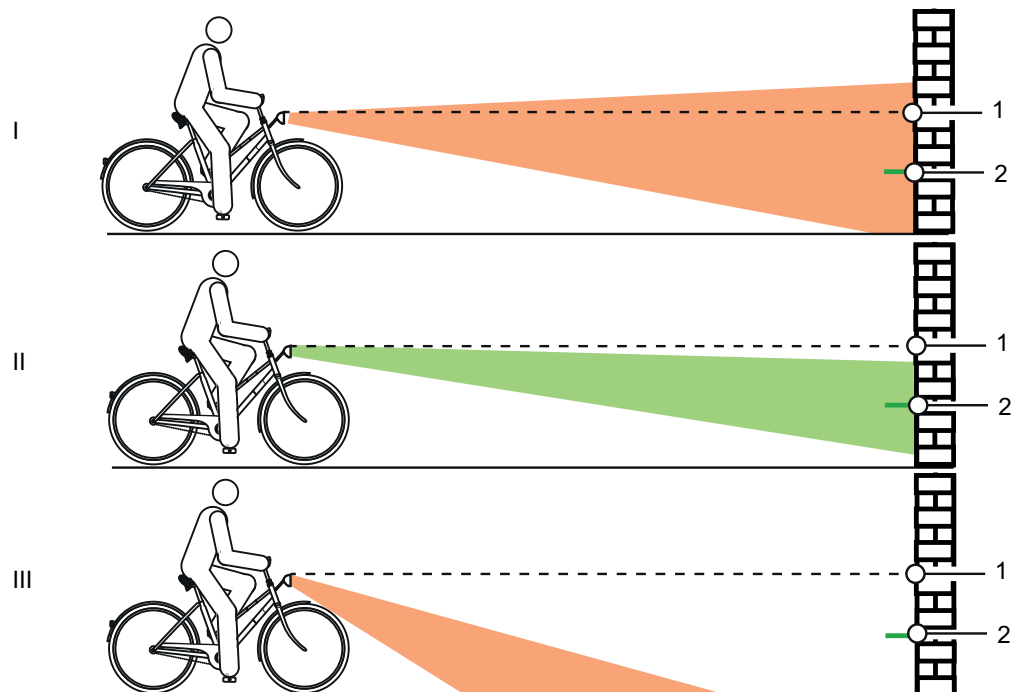
Abbildung 65: Zu hoch (1), korrekt (2) und zu tief (3) eingestelltes Licht
