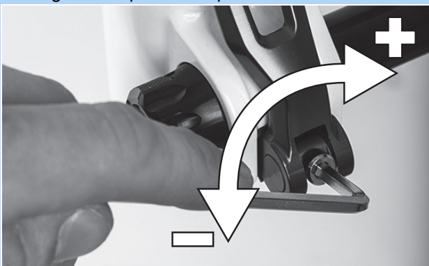
Abbildung 97: Spannkraft des Schnellspanners einstellen
