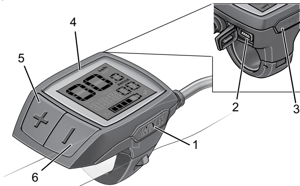
Abbildung 26: Aufbau BOSCH Purion Bordcomputer
