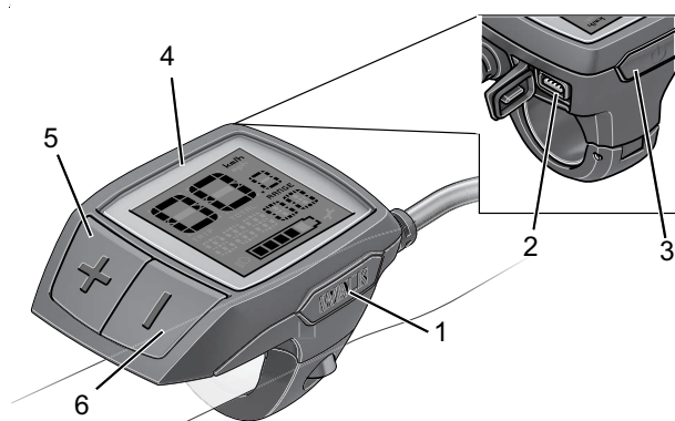
Abbildung 74: Aufbau BOSCH Purion Bordcomputer
