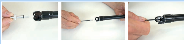
Abbildung 122: Kartusche Ventildeckel befestigen
