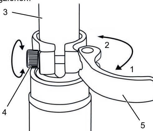
Abbildung 43: Schnellspanner der Sattelstütze öffnen
