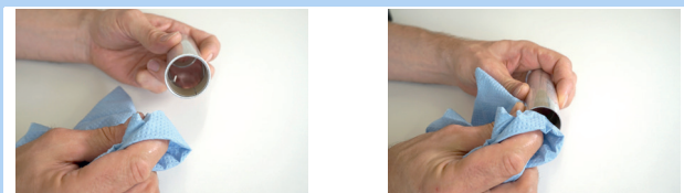
Abbildung 114: Gleitbuchsenrohr reinigen
