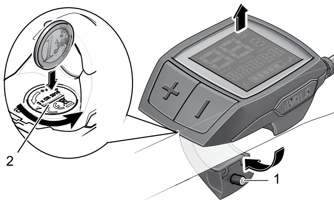
Abbildung 75: Bordcomputer mit Befestigungsschraube (1) und Batteriefachdeckel (2)
