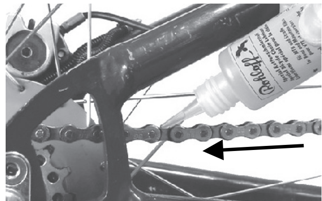
Abbildung 84: Kette schmieren
