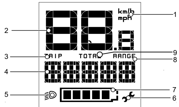
Abbildung 27: Übersicht Bildschirm
