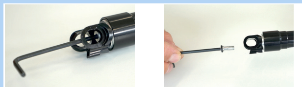
Abbildung 115: Ventilkappe herausdrehen
