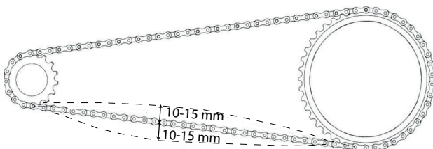
Abbildung 91: Kettenspannung prüfen
