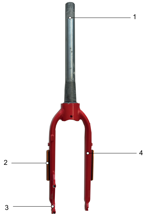
Abbildung 6: Übersicht Gabel
