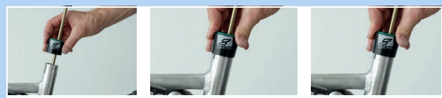
Abbildung 131: Außenhülse aufstecken
