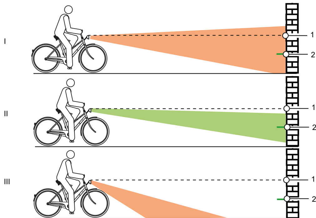
Figur 101: For højt (1), korrekt (2) og for lavt (3) indstillet lys
