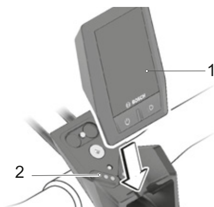
Figur 70: Påsætning af cykelcomputer (1)
