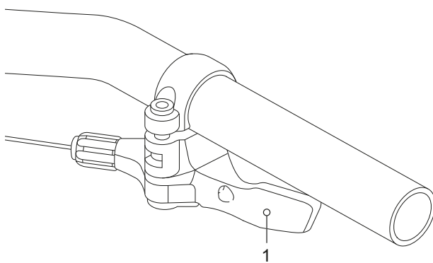
Figur 48: Fjernbetjeningens betjeningsgreb (1)
