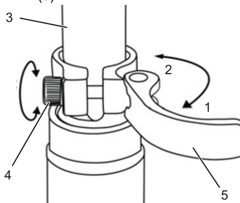
Figur 46: Løsning af sadelpindens hurtigbespænding
