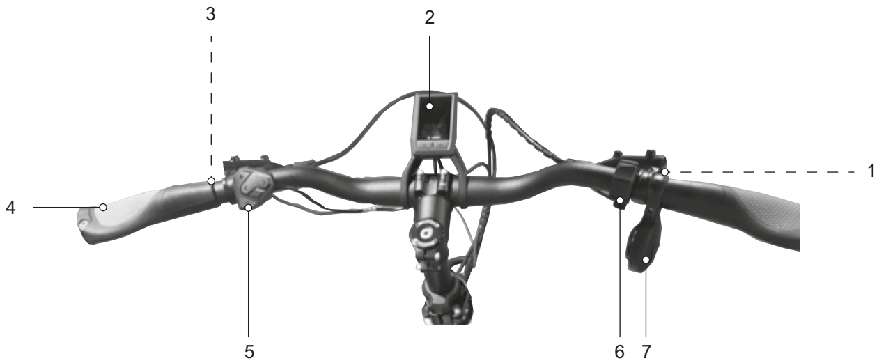
Figur 26: Detaljeret visning styr med BOSCH Kiox-cykelcomputer, eksempel
