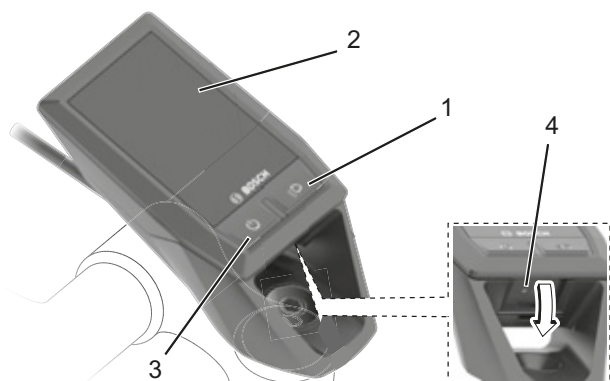
Figur 69: Oversigt over cykelcomputerens opbygning og betjeningslementer
