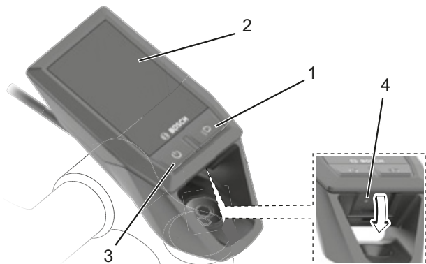
Figur 84: Oversigt over cykelcomputerens opbygning og betjeningsselementer
