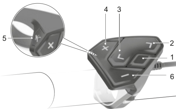
Figur 74: Oversigt over betjeningsenhed
