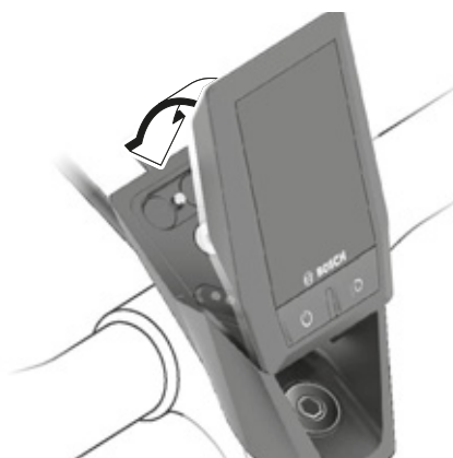
Figur 71: Cykelcomputeren vippes fremad
