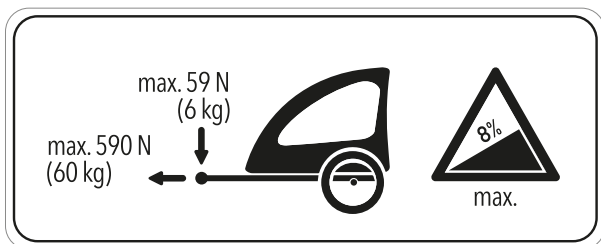
Figur 66: Infoskilt på cykelanhænger
