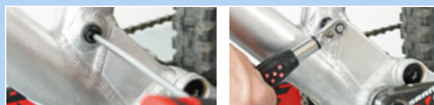
Figur 130: Fastgørelse af postpin-aksel
