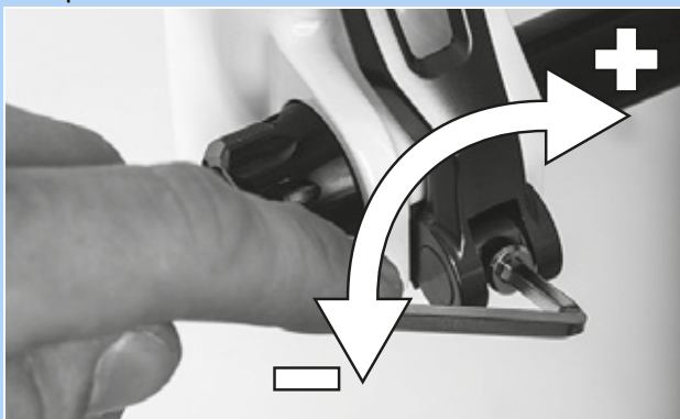
Figur 98: Indstilling af hurtigbespændingens spændekraft
