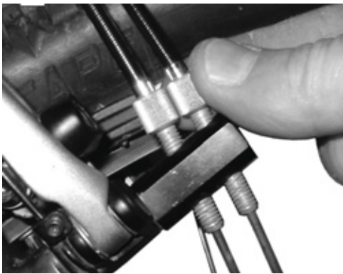
Figur 92: På udgaver af Rohloff-nav med intern skifteaktivering sidder kabelindstilleren på kabelmodholdet
