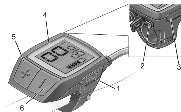
Figur 74: BOSCH Purion-cykelcomputerens opbygning
