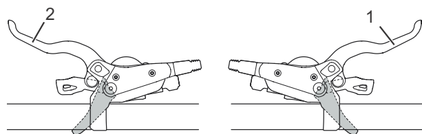
Figur 76: Bremsegreb til bagbremse (1) og forbremse (2), SHIMANO-bremse som eksempel
