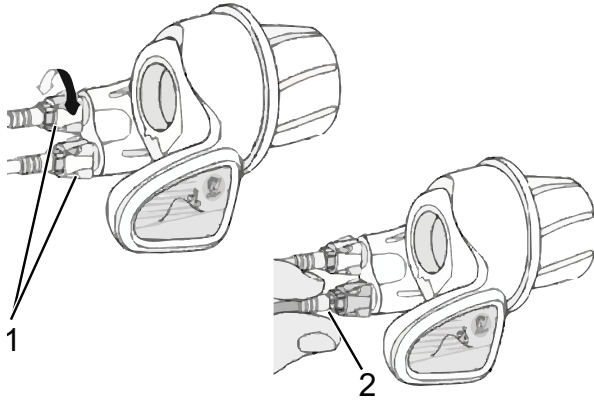
Figur 96: Drejegræb med slutmuffer (1) og gearskiftets slør (2)
