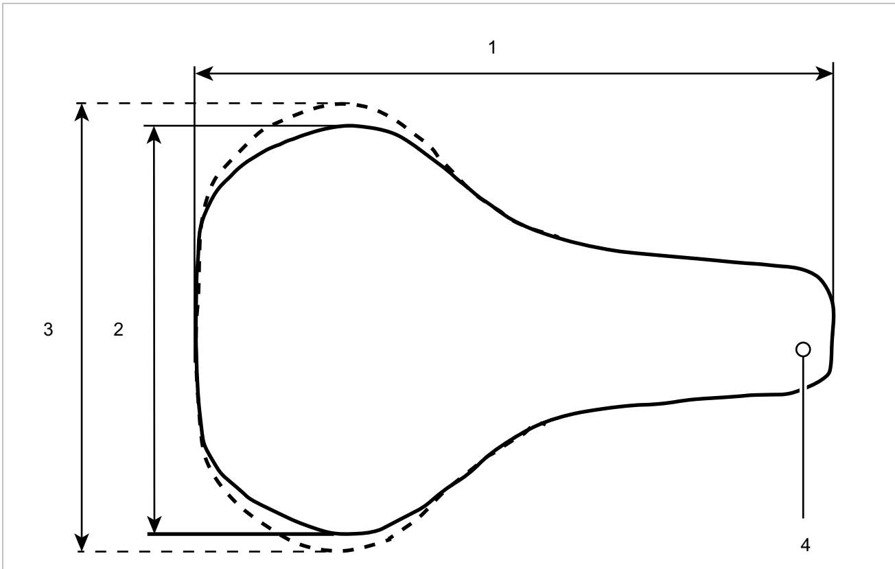
Afbeelding 22: Afmetingen zadel
