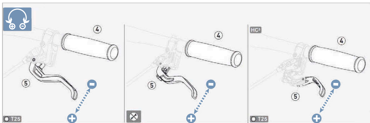
Afbeelding 91: Grijpafstand handrem MAGURA schijfrem afstellen
