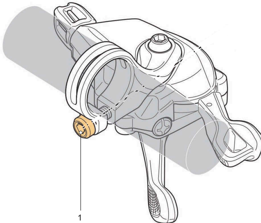
Afbeelding 93: Locatie bevestigingsschroef (1)
