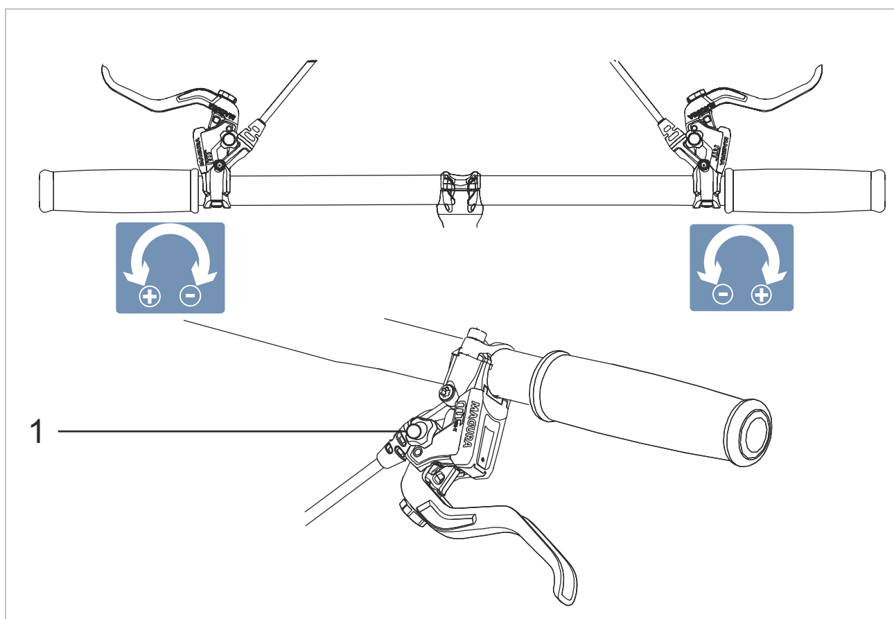
Illustration 92 : Utilisation du bouton rotatif (1) pour le réglage du point de pression
