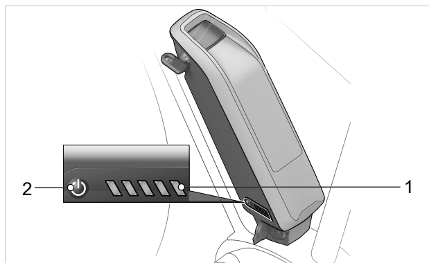
Illustration 53 : Position de l'indicateur de charge de la batterie pour tube de selle
