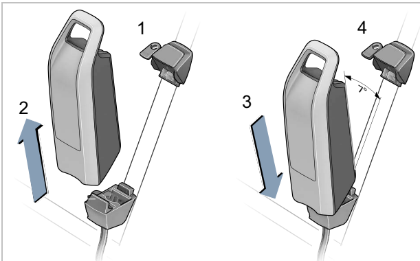
Illustration 116 : Retirer et insérer la batterie sur cadre
