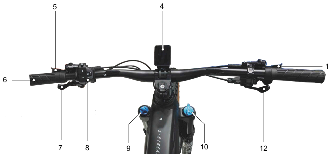
Illustration 39 : Vue détaillée du guidon avec ordinateur de bord FIT Remote Basic et écran Compact 2.0, exemple
